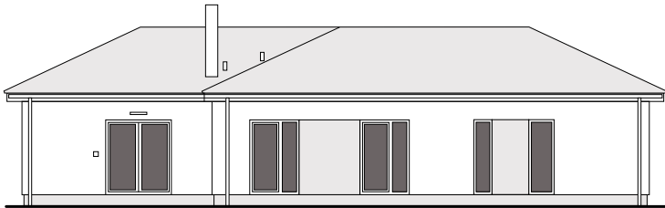
POHLED P3
