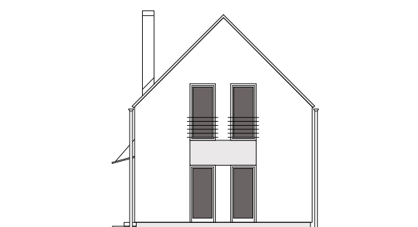
POHLED P4
