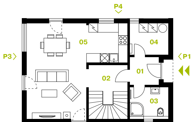
PŮDORYS PŘÍZEMÍ
