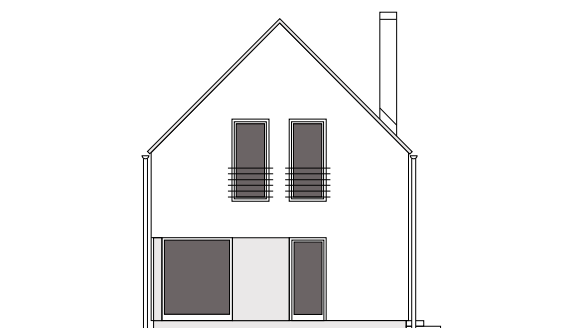
POHLED P3
